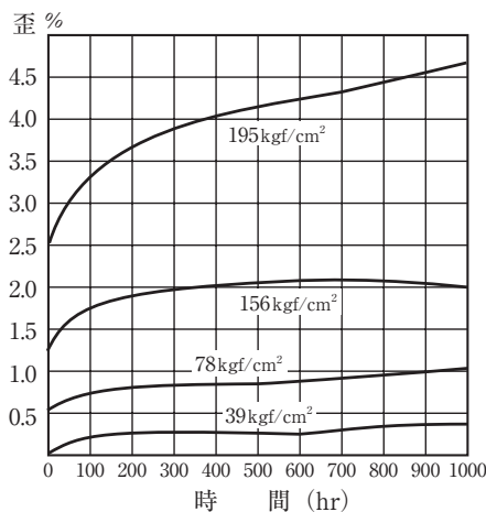
ポリカーボネートのクリープ (100°C)
