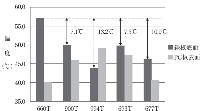
屋外施工試験 温度比較 (12:00～15:00 平均温度)
