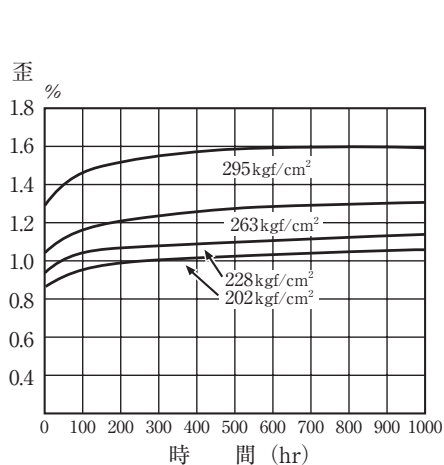
ポリカーボネートのクリープ (23°C)
