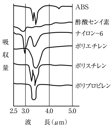
熱可塑性プラスチックの熱線吸収曲線
